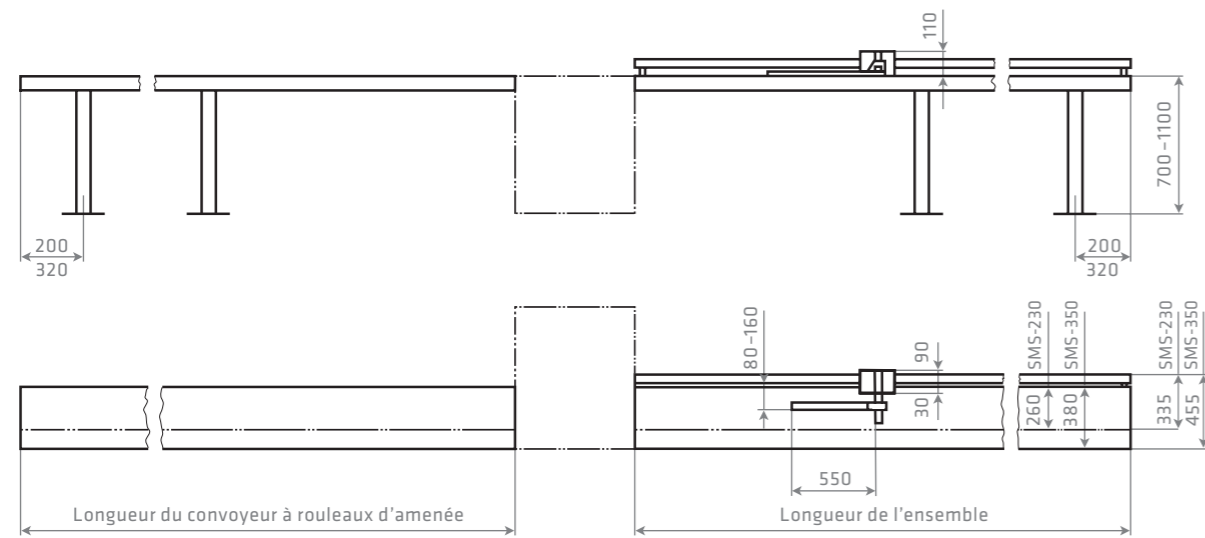
Convoyeur à rouleaux d'amenée ZFB
