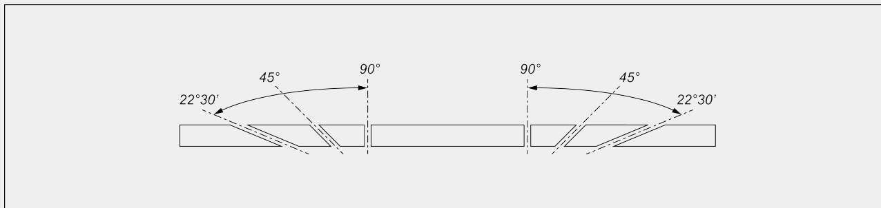
Réglage mécanique des angles intermédiaires
